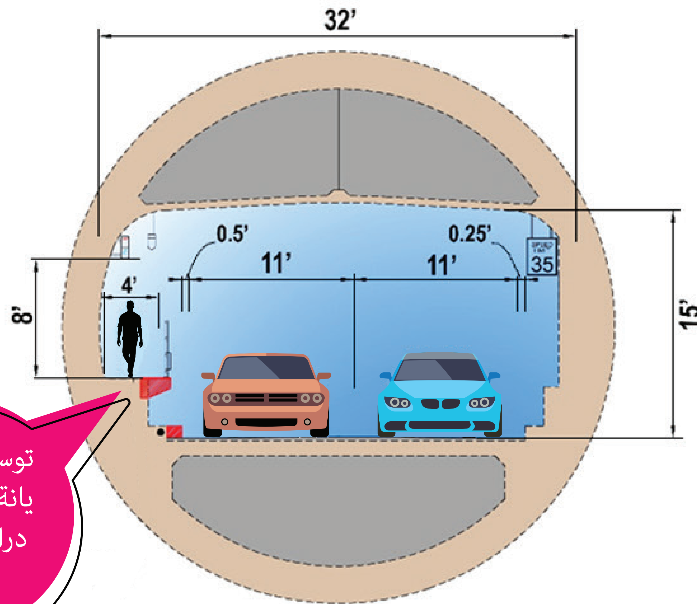
Webster المقطع العرضي لنفق
