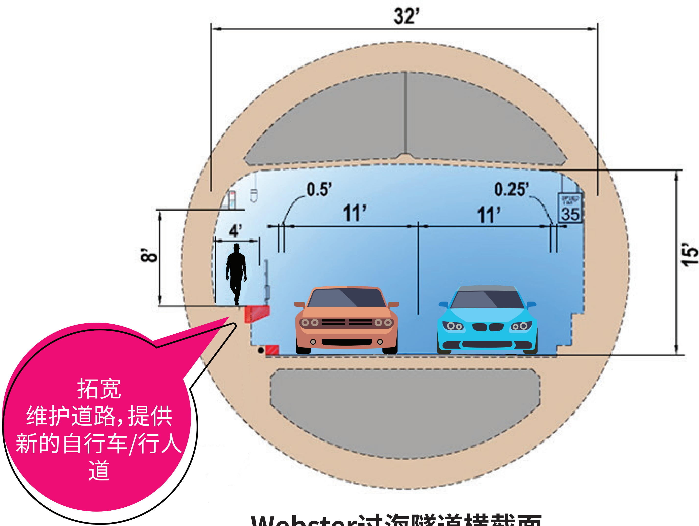
Webster过海隧道横截面
