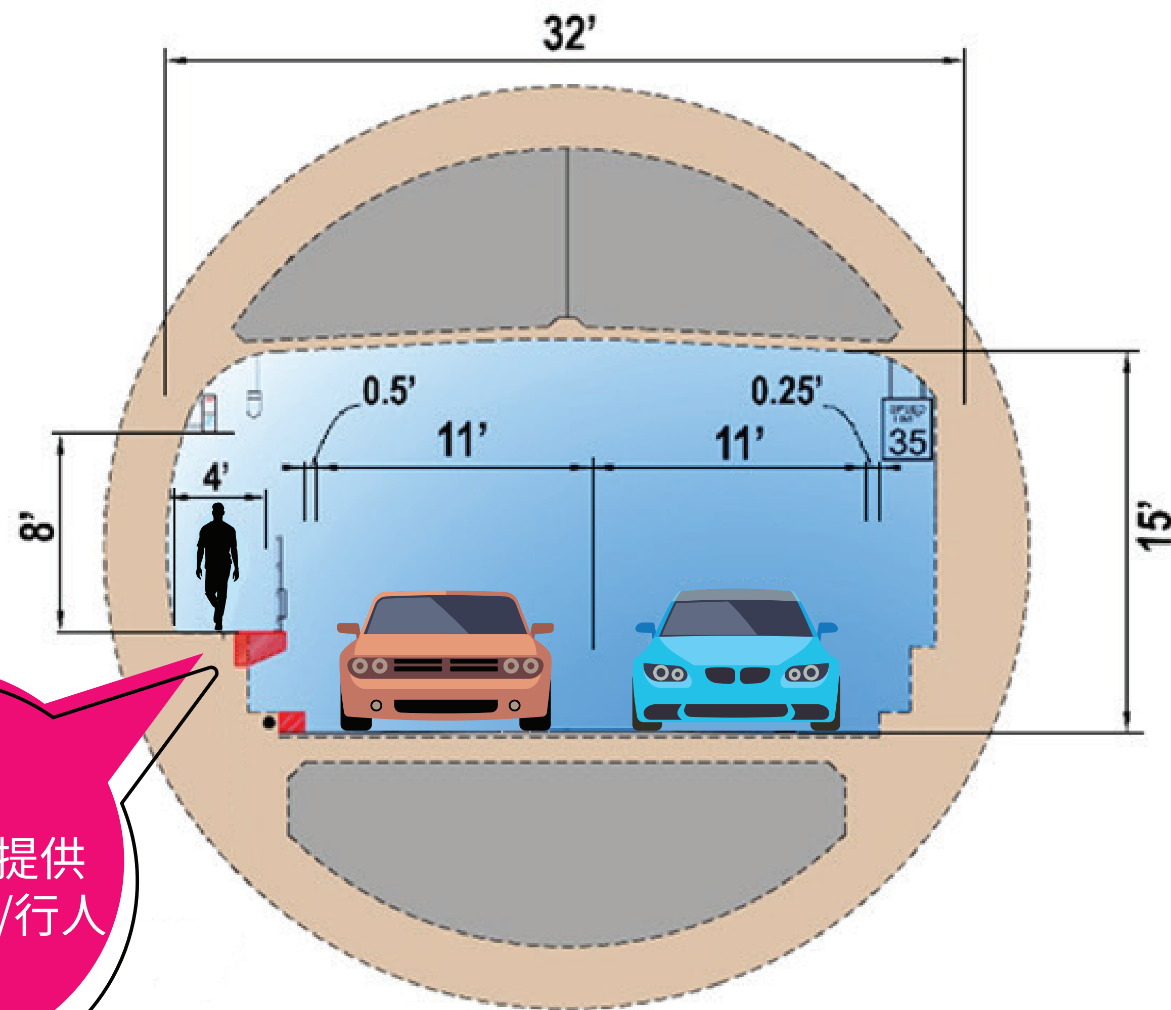
Webster过海隧道横截面
