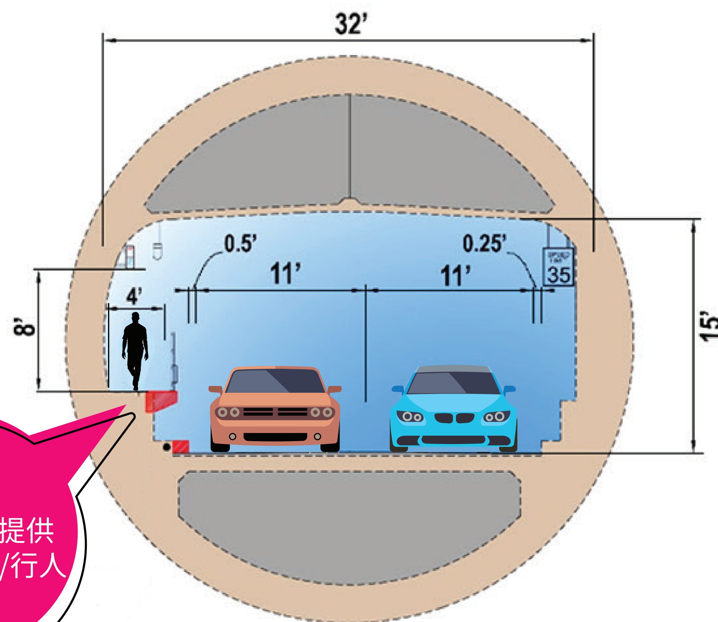
Webster過海隧道橫斷面
