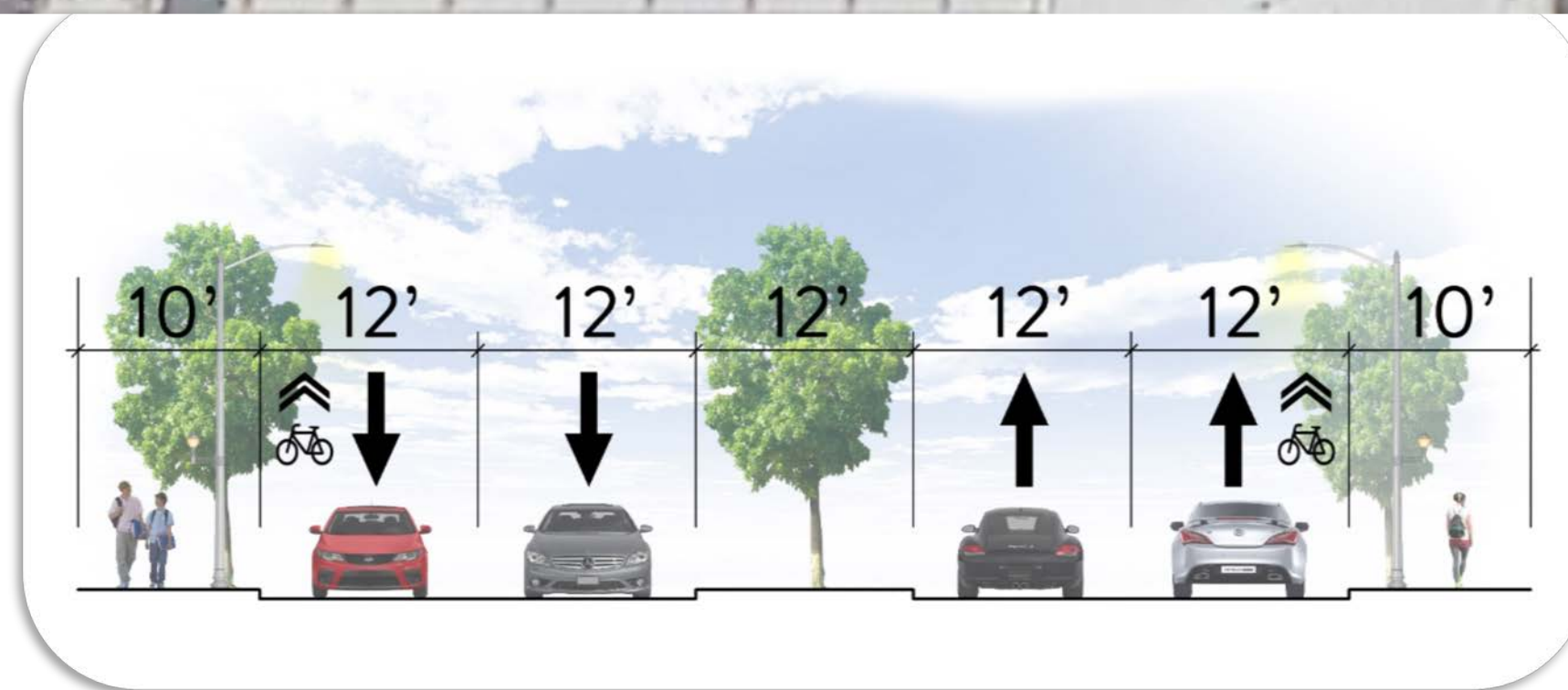
SECTION D-D
